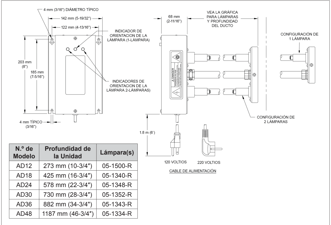
Figura 2 – Datos Dimensionales en mm (pulgadas), m (pies)
