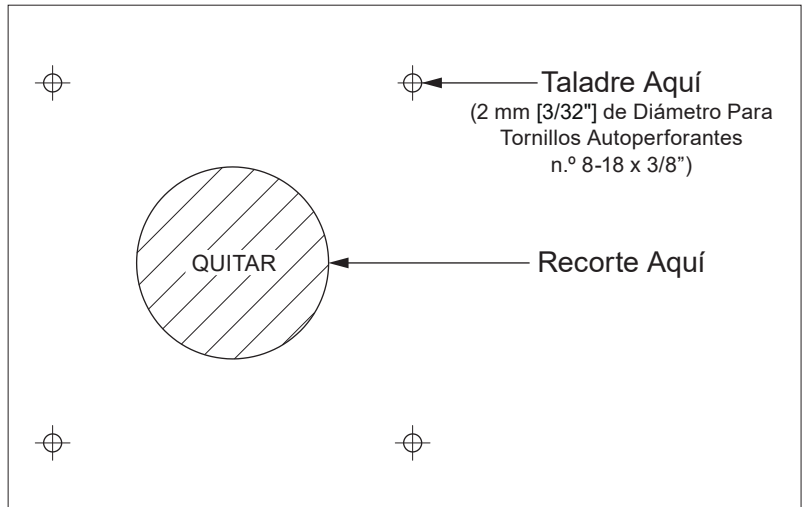
Figura 4 – Escala Real Plantilla de Montaje del Lente Visor 25mm (1")
