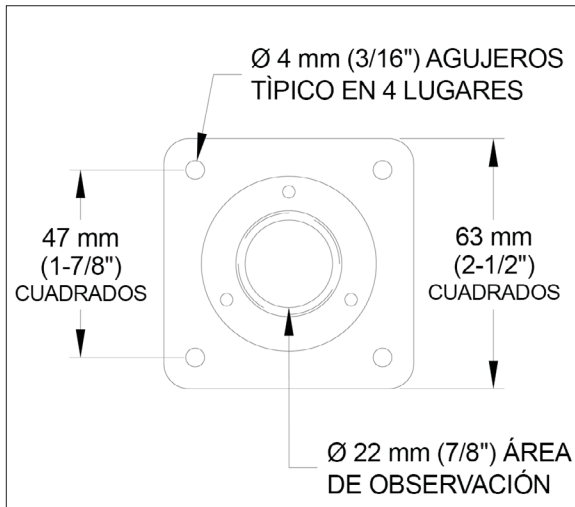
Figura 3 – Datos Dimensionales del Lente Visor Promate™
