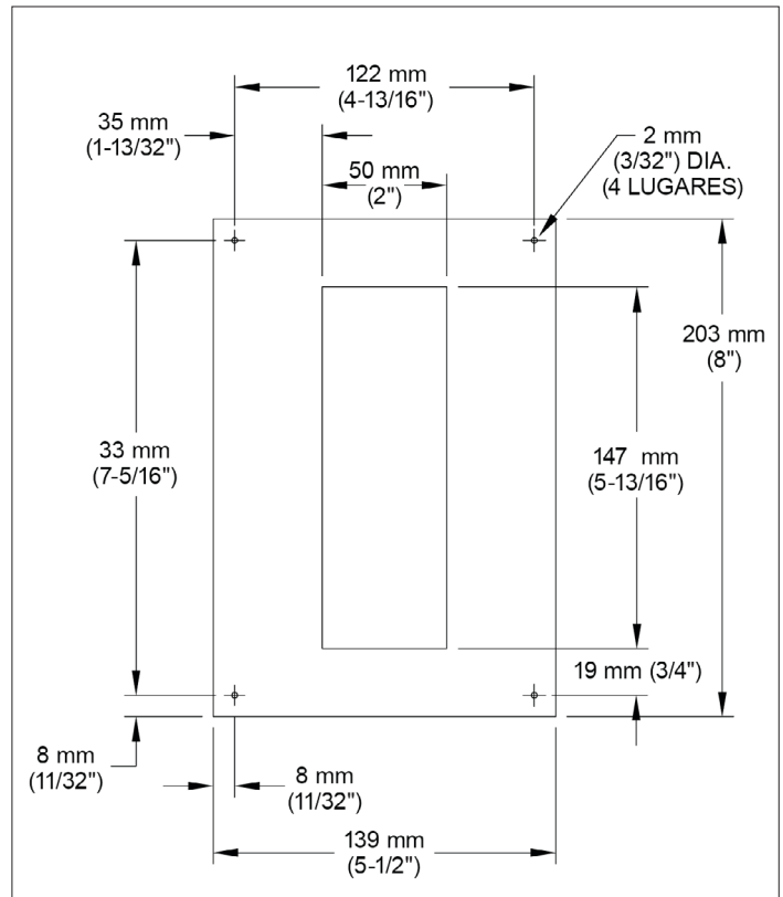
Figura 6 – Plantilla de Montaje Datos Dimensionales AD (2 Lámparas)
