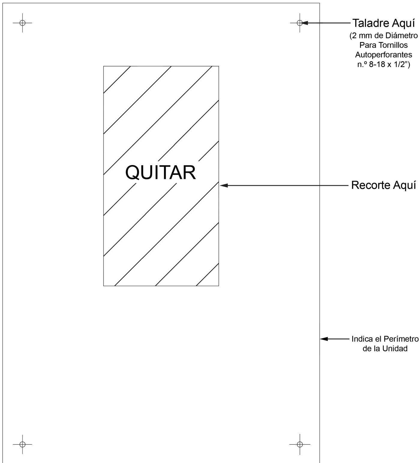
Figura 7 – Plantilla de Montaje AD - A Escala Real (1-Lámpara)
