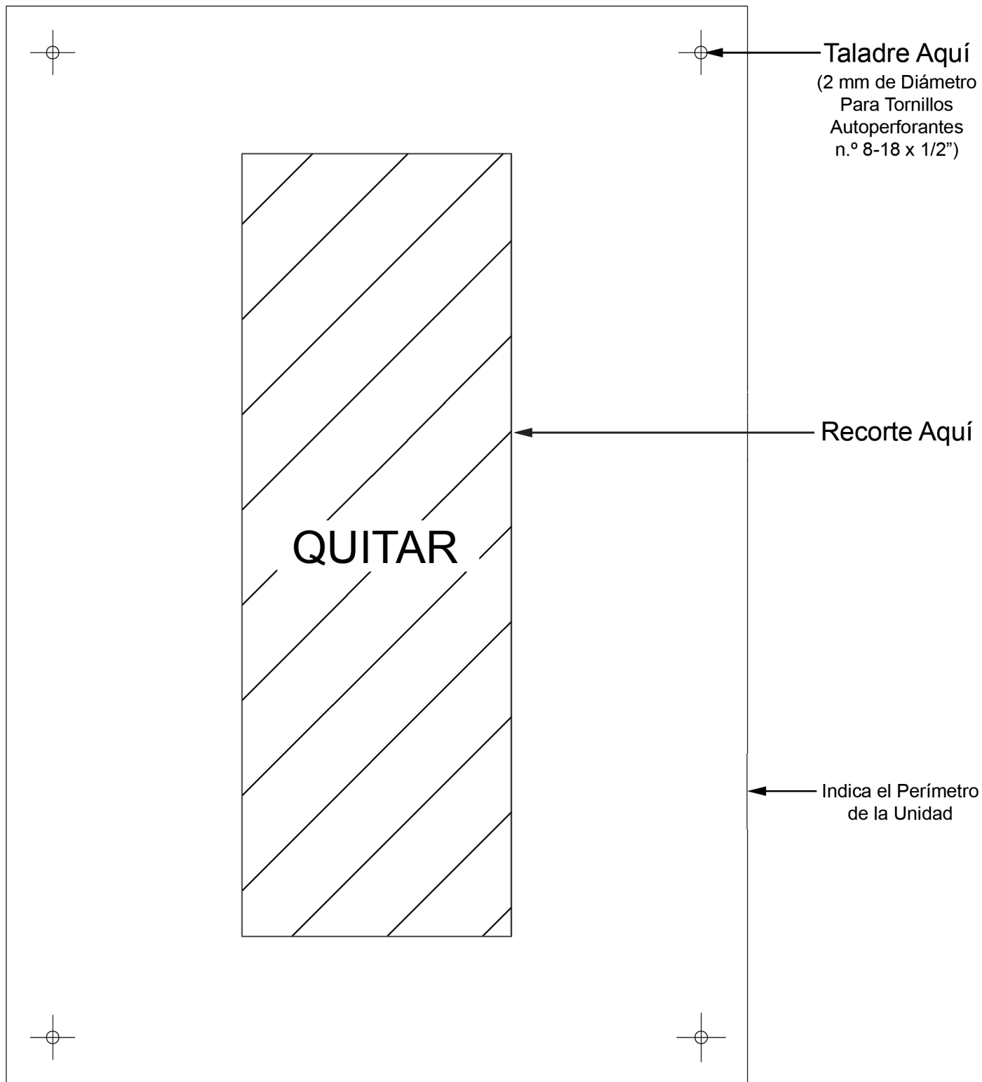
Figura 8 – Plantilla de Montaje AD - A Escala Real (2-Lámpara)
