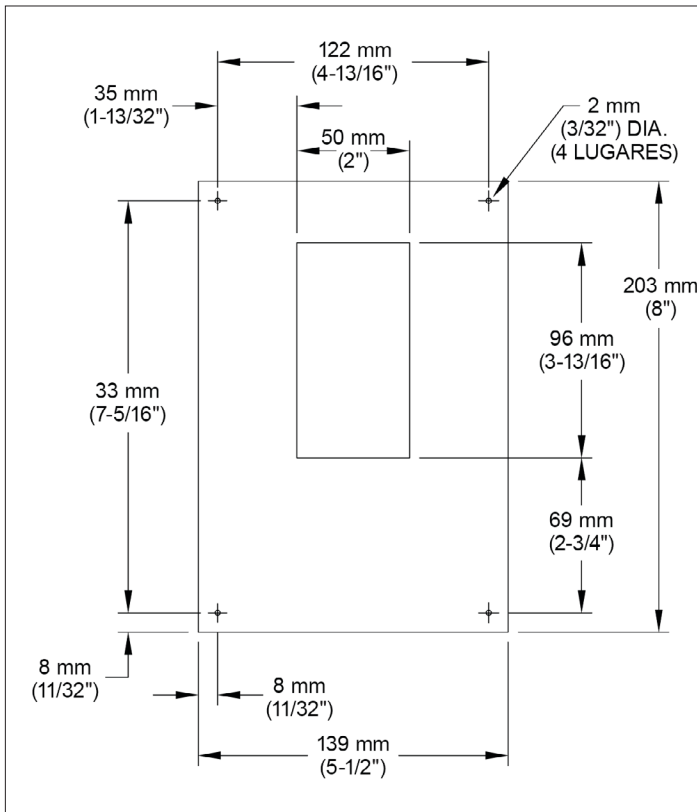
Figura 5 – Plantilla de Montaje Datos Dimensionales AD (1 Lámpara)
