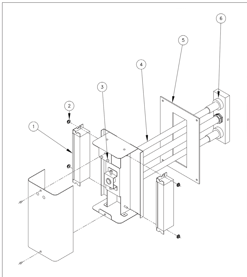
Figura 8 – Vista Explotada (AD18-2)
